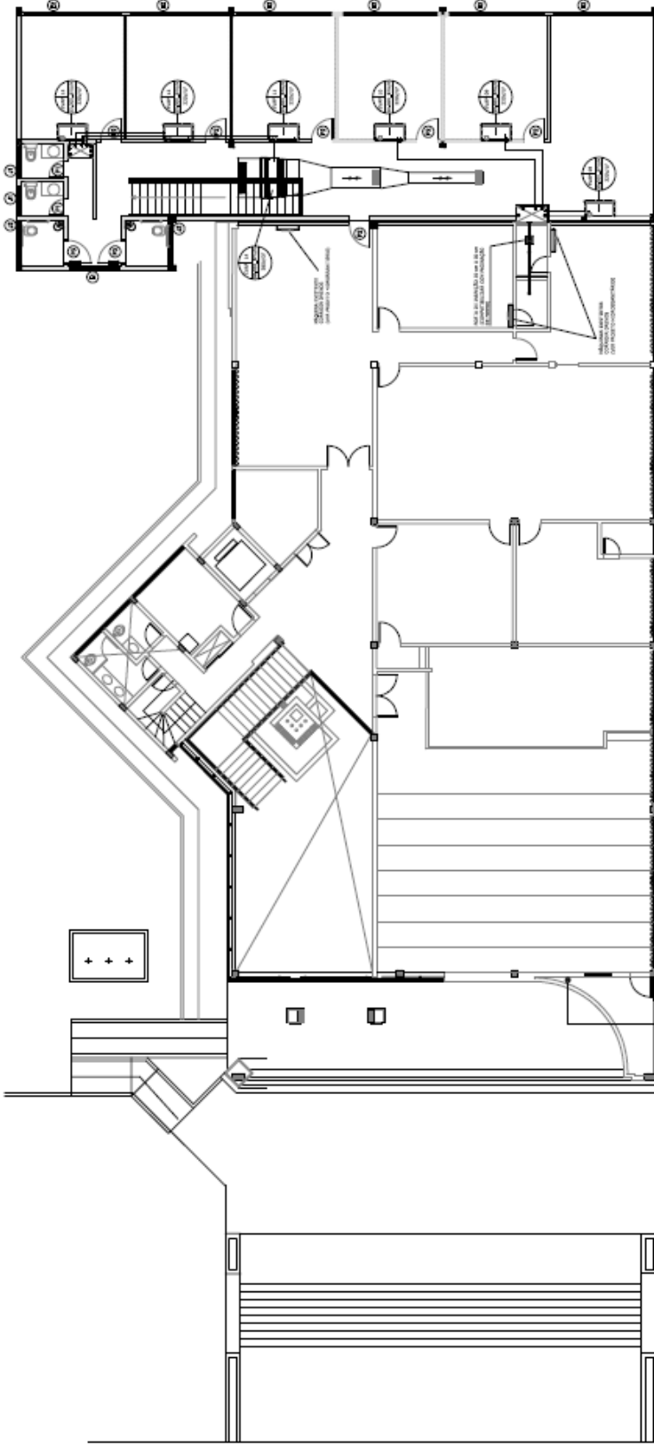
PAVIMENTO SUPERIOR - UNIDADES EVAPORADORAS/DUTOS DE AR/TUBULAÇÃO DE DRENO
