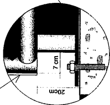
Detalhe Fixação 2
