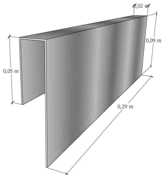
01 PROTÓTIPO PLACA INOX SEM ESCALA
