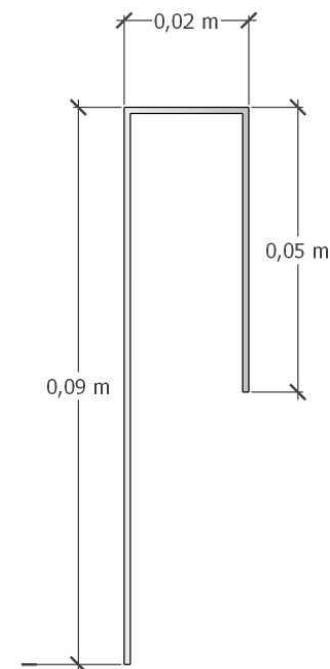
02 PLACA INOX - CORTE SEM ESCALA
